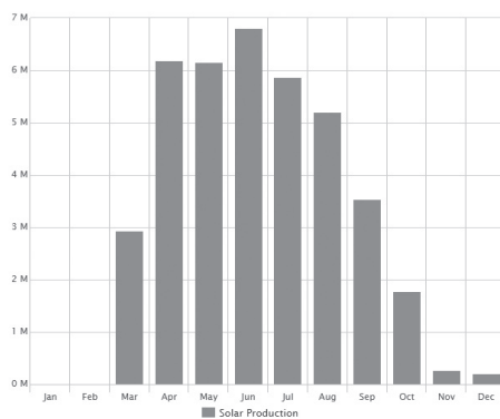
Elproduktionen vid Linköpings missionskyrkas solcellssystem från 9 mars till 31 december 2019. Den högsta stapeln för månaden juni är nästan 7000 kWh hög.
