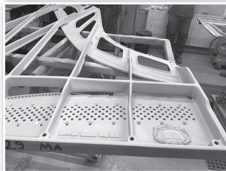
Renoveringen av Missionskyrkans nya flygel pågår just nu i Polen. Bl.a. har järnramen (nedre bilden) lackats om.
